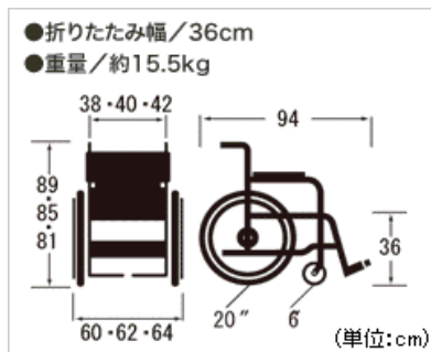
自走式・低床タイプ
