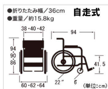
自走式・ 低床タイプ
